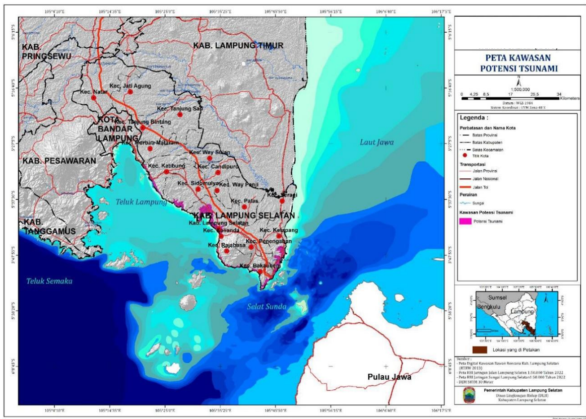
Gambar II.26 Peta Potensi Tsunami Kabupaten Lampung Selatan
