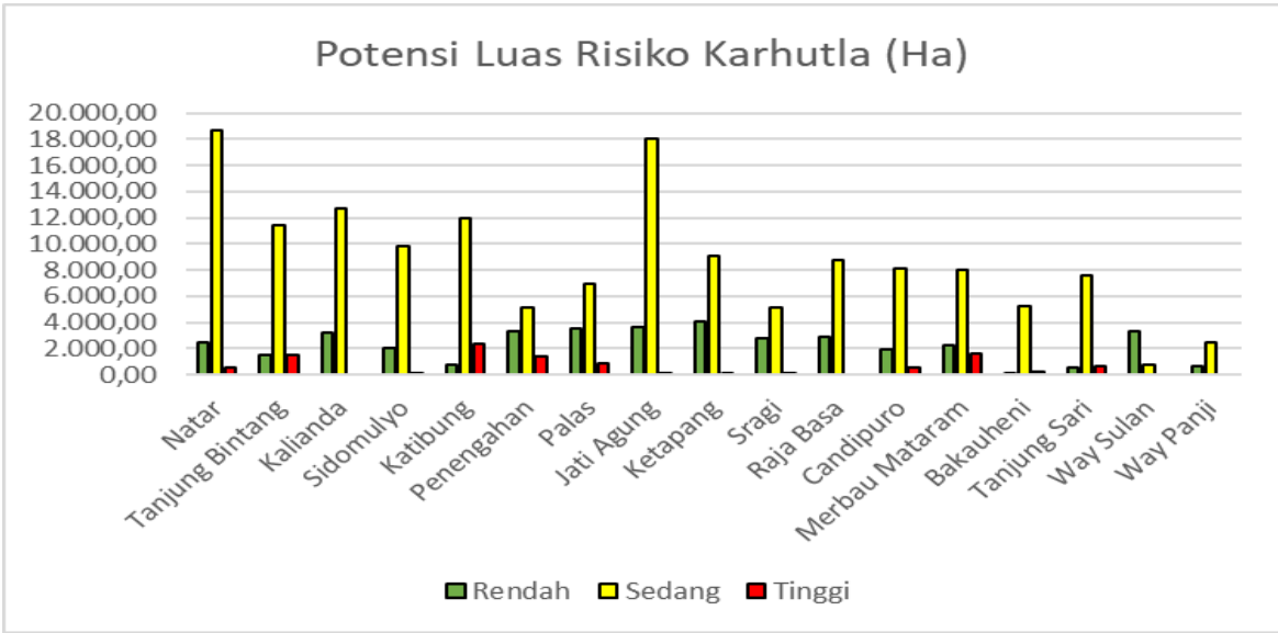
Gambar II.35 Potensi Luas Risiko Karhutla
